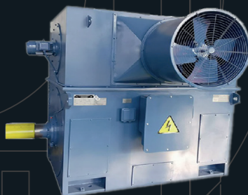
Motores de alta-media tensión aptos para variación de frecuencia
