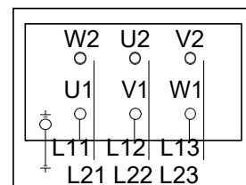
Conexión para arranque estrella-triángulo
