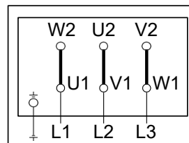
Conexión Delta
