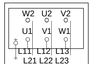
Conexión para arranque estrella-triángulo
