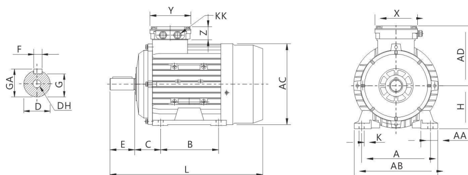
Montaje B3 con patas sin Flanche
