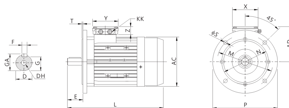
Montaje sin patas y brida B5
