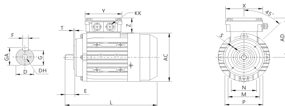
Montaje sin patas y brida B14
