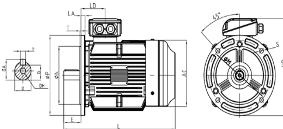
Montaje sin patas y brida B5
